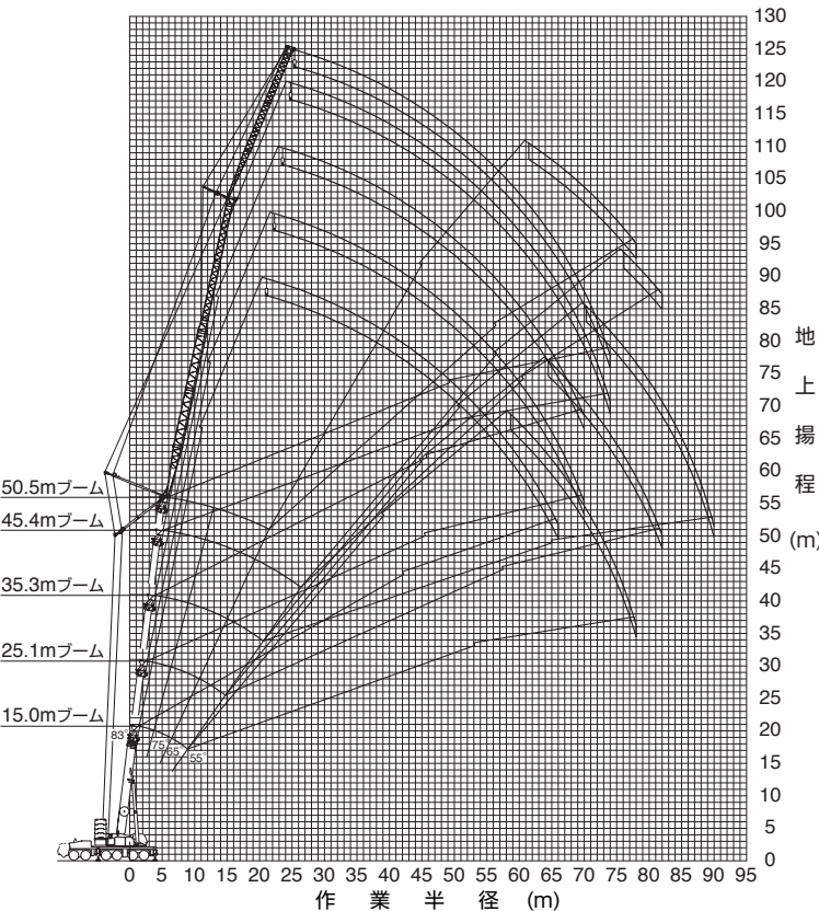
2.1m+47mラフィングジブ+25mエクステンションジブ
