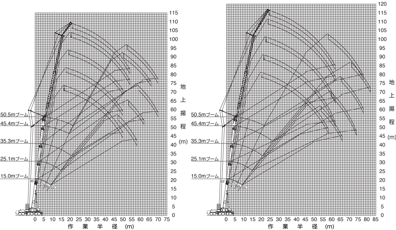
2.1m+47mラフィングジブ+9mエクステンションジブ 2.1m+47mラフィングジブ+17mエクステンションジブ
